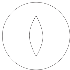
50cm Durchmesser 10x30cm Schlitz
